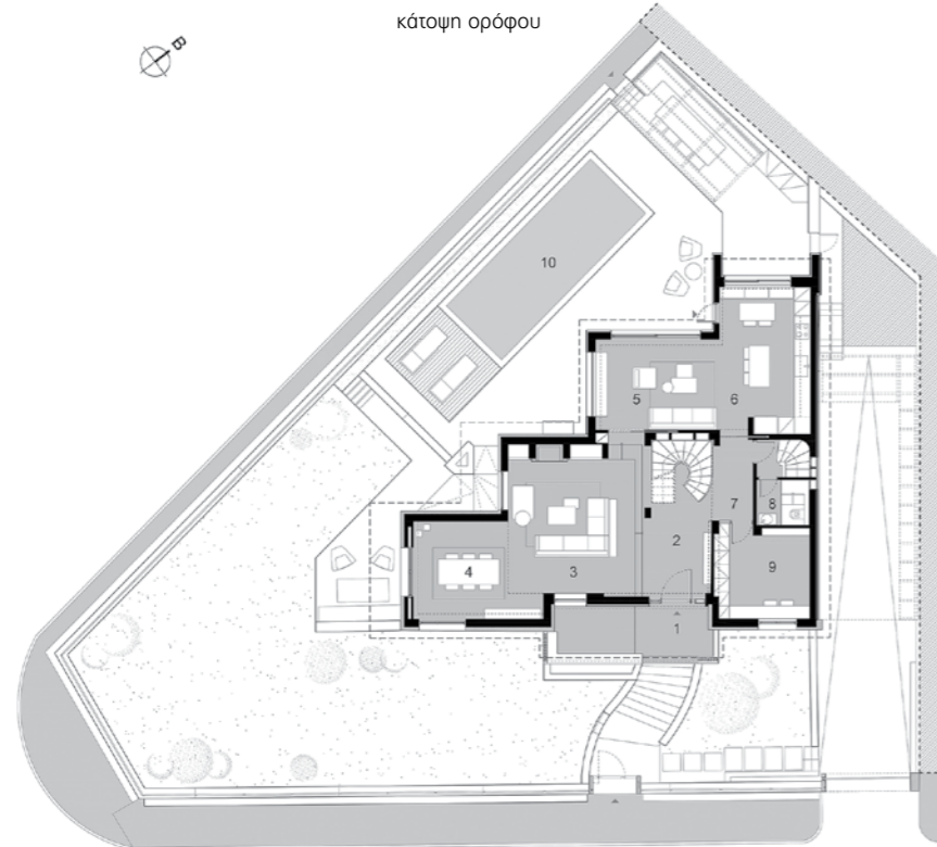
κάτοψη ισογείου
